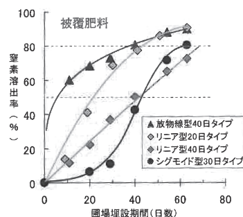
図2 被覆肥料の溶出パターン
