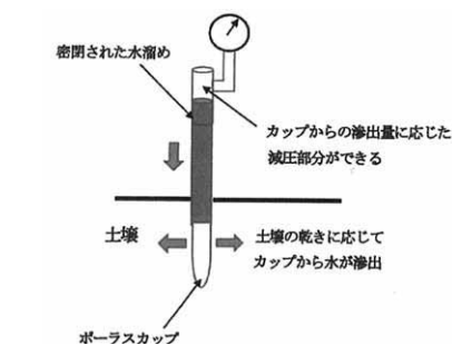
図1 テンシオメータの原理
